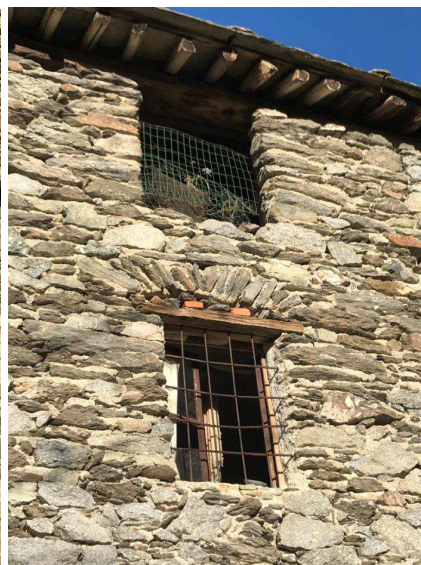
Figura 46: piattabanda in conci di pietra
